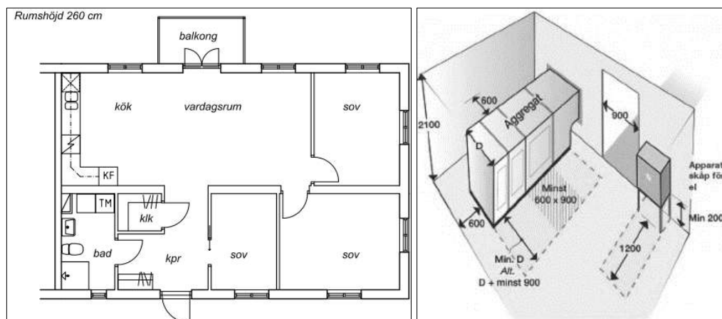
Planlösning lägenhet
